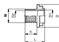
MANICOTTO PER AGITATORE MIXER COUPLING RÜHRWERKANSCHLUß
