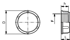
TAPPO FEMMINA BLANKING STOPFEN MIT INNENGEWINDE
