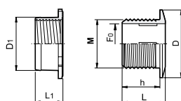
RACCORDO LIVELLO ATOMIZZATORE (2 PEZZI) ATOMISER LEVEL FITTING (2 PIECES) VERBINDUNGSSTÜCK FÜR SPRÜHGERÄTTUNNEL (2 STÜCKE)
