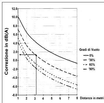
GRAFICO CORREZIONE RUMORE KTS
