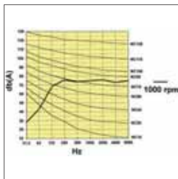
KTM 2300
