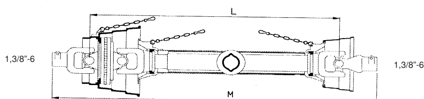
ALBERI CARDANICI OMOCINETICI GRANDANGOLARI. 1 GIUNTO OMOCINETICO LATO TRATTORE WIDEANGLE CV PTO DRIVE SHAFTS WITH 1 CV JOINT AT TRACTOR SIDE WEITWINKEL-GLEICHLAUF-GELENKWELLEN MIT 1 WEIß GELENK SCHLEPPER SEITIG
